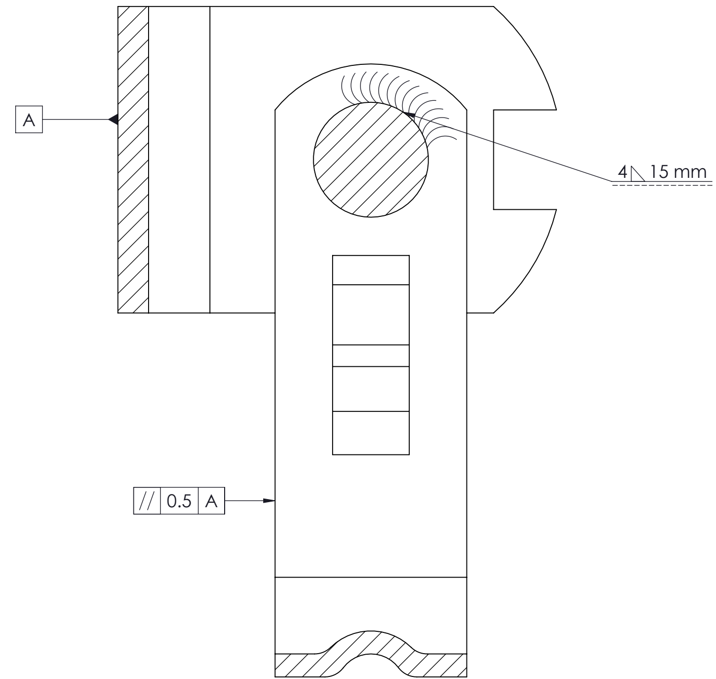
DOORSNEDE A-A SCHAAL 2:1
