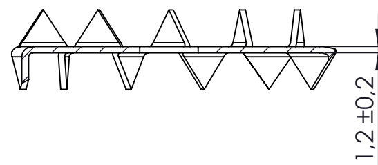
DOORSNEDE A-A
