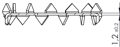
DOORSNEDE A-A
